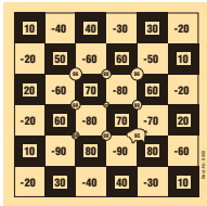
Schachbrett
