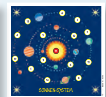
Sonnensystem
