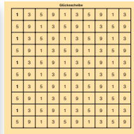
Zahlenfelder
